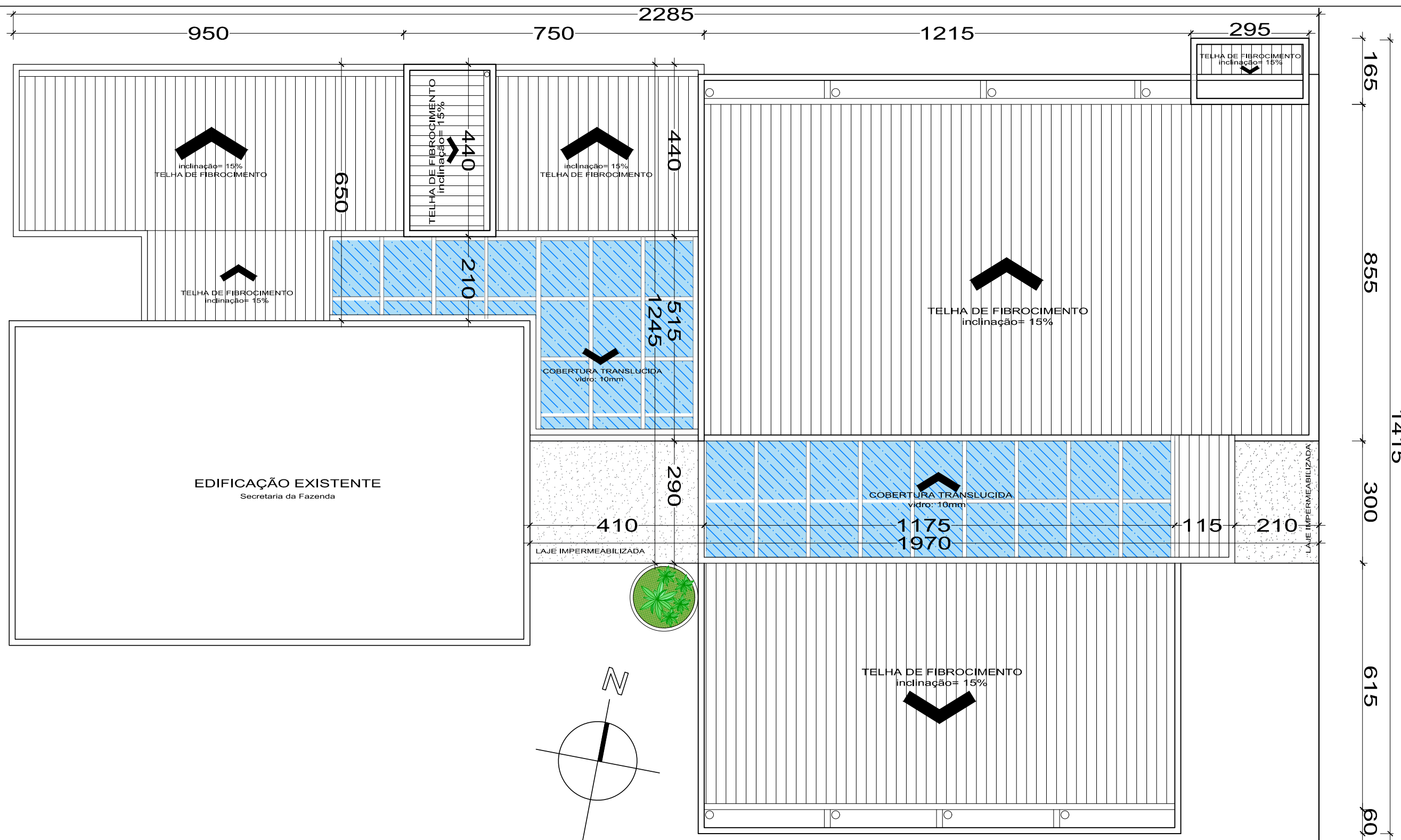
PLANTA DE COBERTURA Escala 1/100
